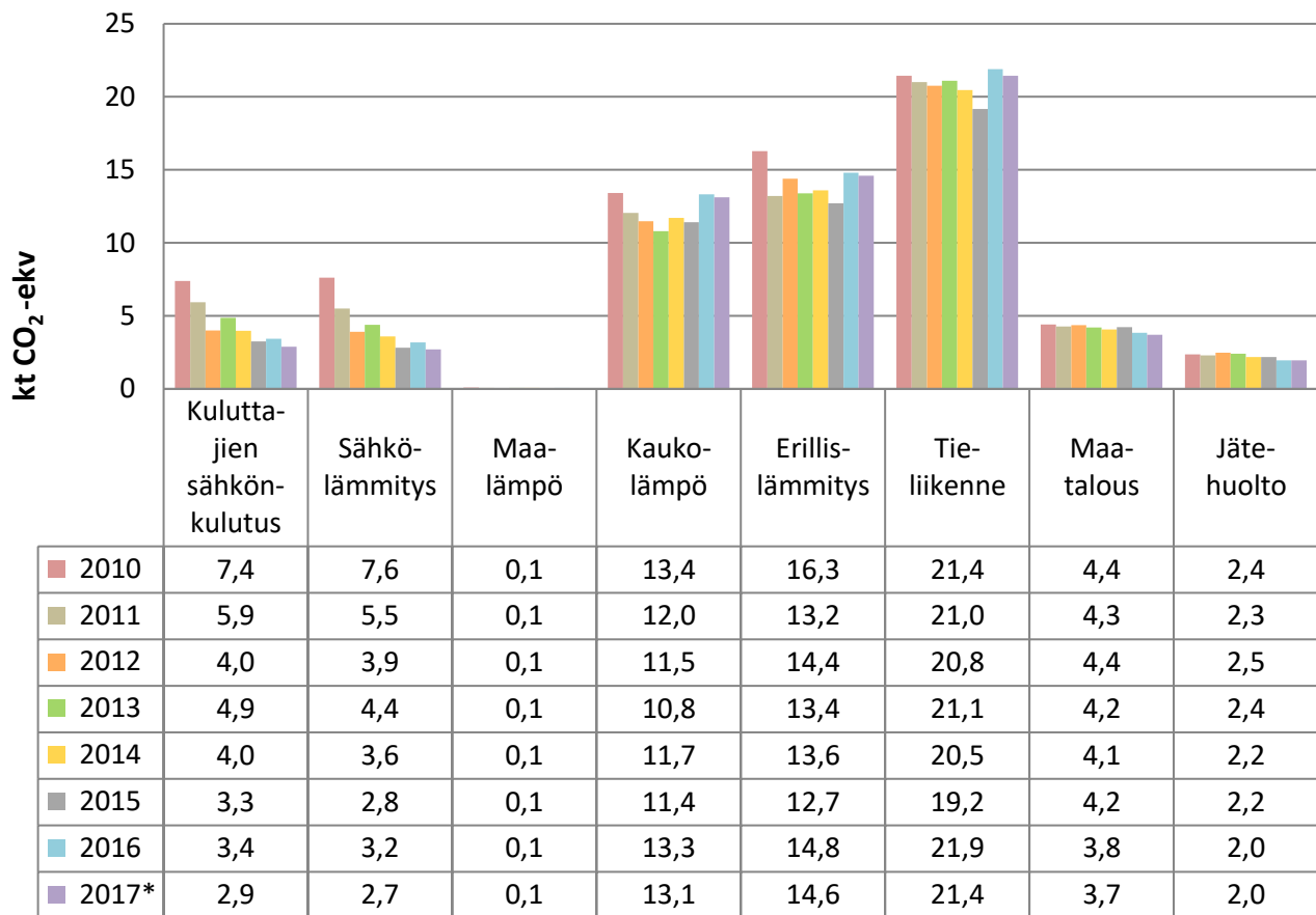
Kuva 15. Päästöt sektoreittain Karkkilassa vuosina 2010–2017 ilman teollisuutta. Vuoden 2017 tieto on ennakkotieto.
