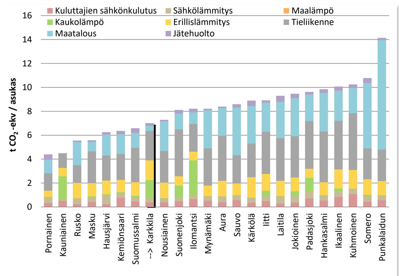
Kuva 19. CO2-raportissa mukana olevien alle 10 000 asukkaan kuntien asukaskohtaiset päästöt vuonna 2016 ilman teollisuutta.
