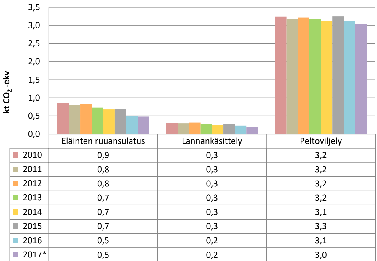
Kuva 10. Maatalouden päästöjen kehitys Karkkilassa vuosina 2010–2017 jaettuna eläinten ruuansulatuksen, lannankäsittelyn ja peltoviljelyn päästöihin.
