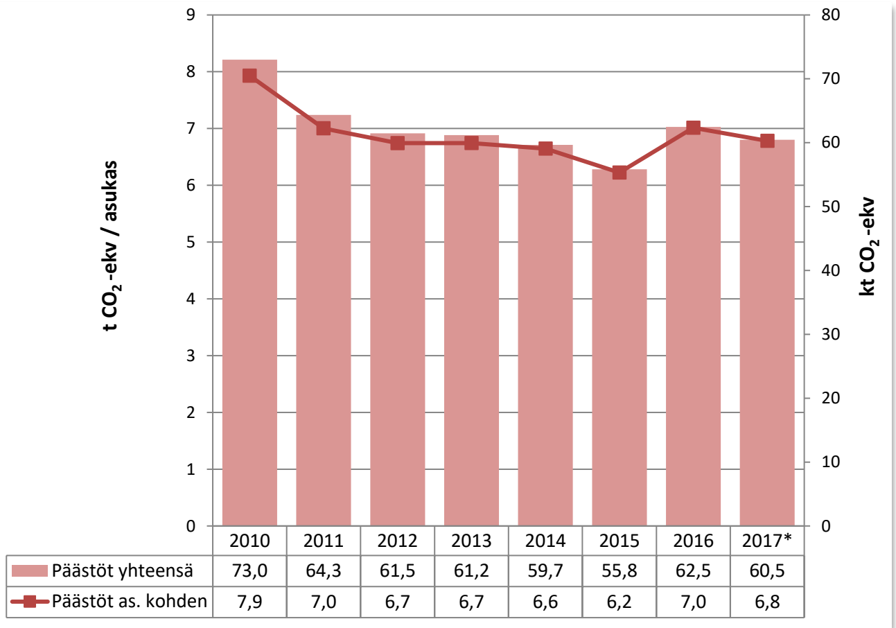
Kuva 16. Päästöt yhteensä ja asukasta kohden Karkkilassa vuosina 2010–2017 ilman teollisuutta. Vuoden 2017 tieto on ennakkotieto.
