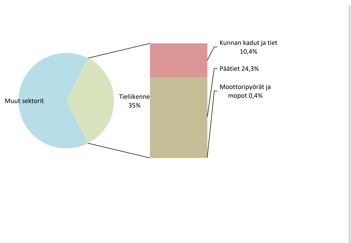
Kuva 7. Tieliikenteen päästöjen osuus kokonaispäästöistä (ilman teollisuutta) Karkkilassa vuonna 2016 ja sektorin jakautuminen eri päästölähteisiin.
