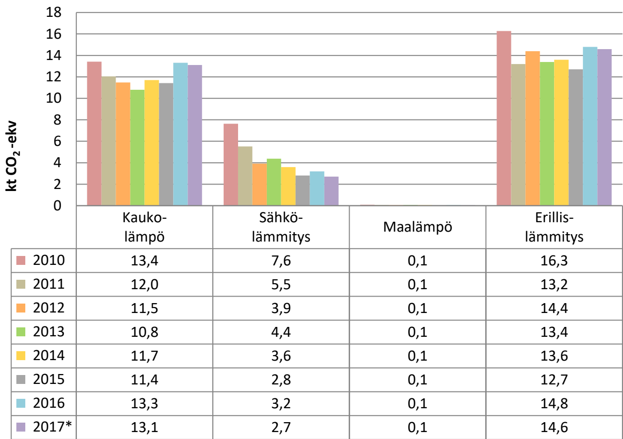
Kuva 6. Rakennusten lämmityksen päästöjen kehitys Karkkilassa vuosina 2010–2017. Vuoden 2017 tieto on ennakkotieto.
