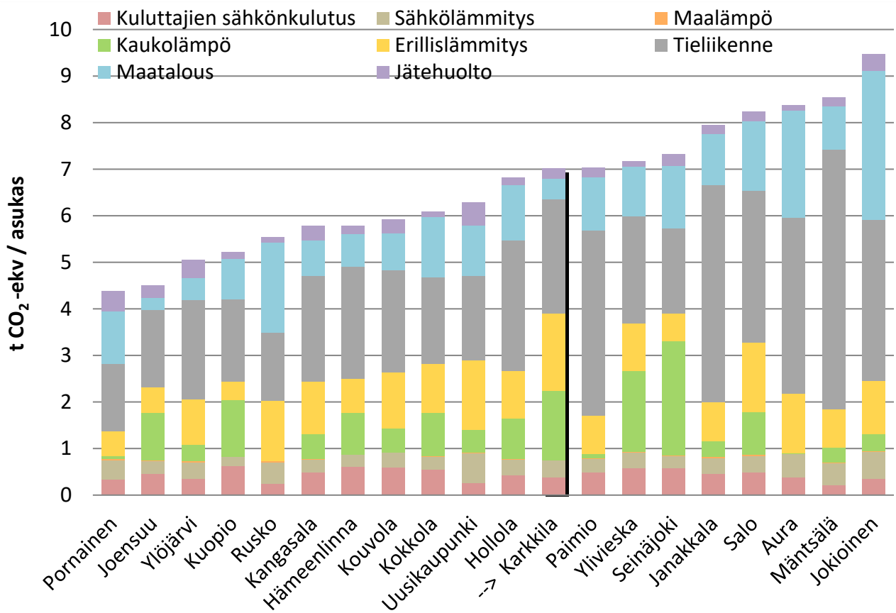
Kuva 20. Asukaskohtaisten päästöjen vertailu (ilman teollisuutta) vuonna 2016 sellaisissa CO2-raportin kunnissa, joissa on 25–50 asukasta maaneliökilometrillä.
