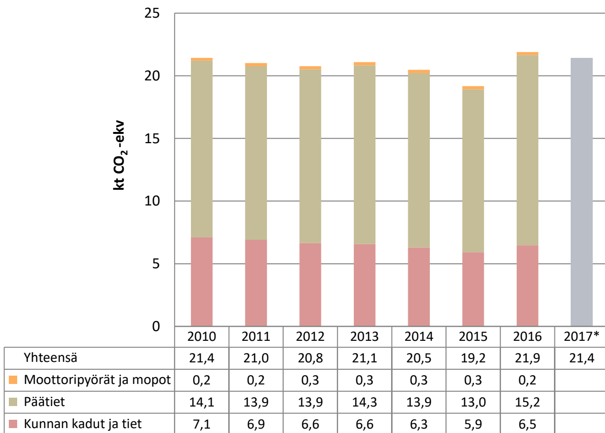
Kuva 8. Tieliikenteen päästöt Karkkilassa vuosina 2010–2017. Vuoden 2017 tieto on ennakkotieto, joka perustuu liikennemäärien muutoksiin kunnan alueella.
