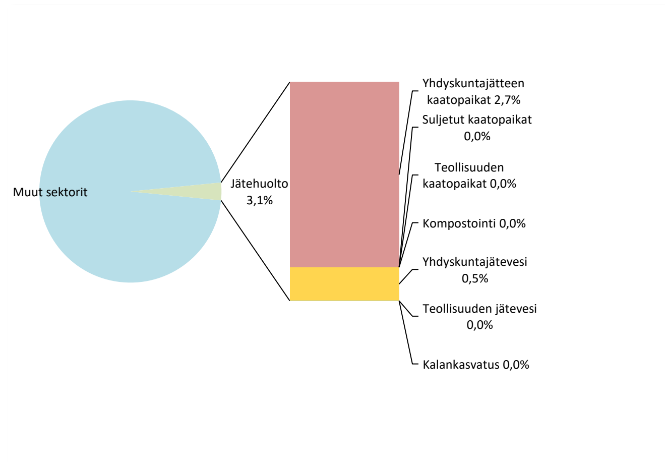
Kuva 11. Jätehuollon päästöjen osuus kokonaispäästöistä (ilman teollisuutta) Karkkilassa vuonna 2016 ja sektorin jakautuminen eri päästölähteisiin.
