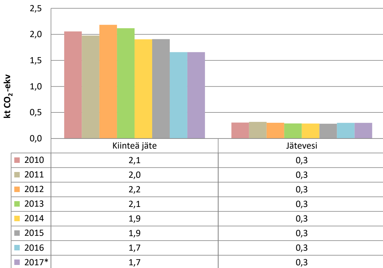
Kuva 12. Jätehuollon päästöjen kehitys Karkkilassa vuosina 2010–2017. Vuoden 2017 ennakkotietona on vuoden 2016 tieto.
