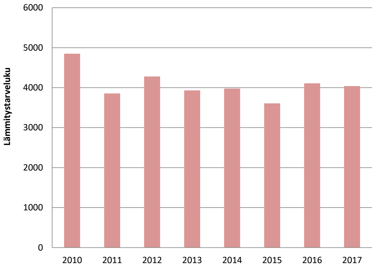
Kuva 4. Karkkilan lämmitystarveluvut vuosina 2010–2017.
