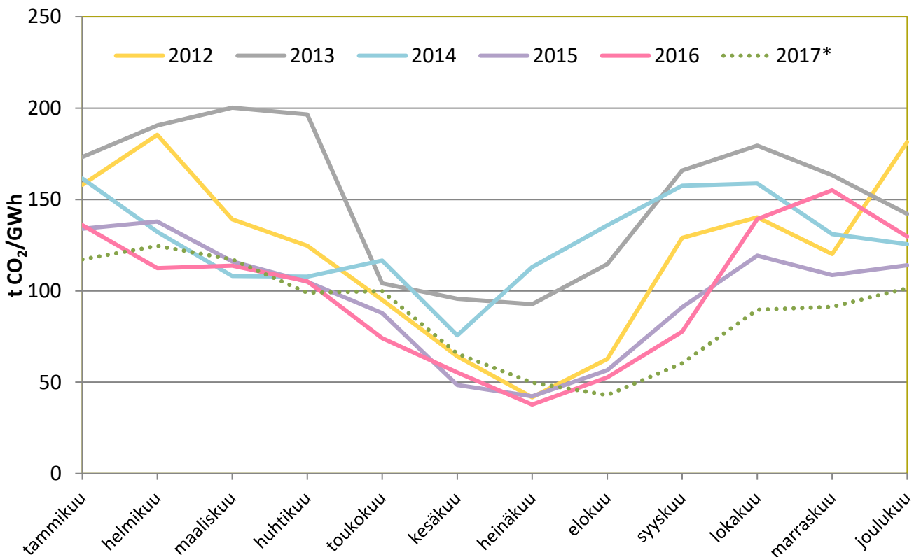
Kuva 1. Sähkönkulutuksen päästökertoimen kuukausitasolla vuosina 2012–2017, laskettuna hyödynjakomenetelmällä Energiateollisuus ry:n aineistosta. Vuoden 2017 tieto on ennakkotieto.
