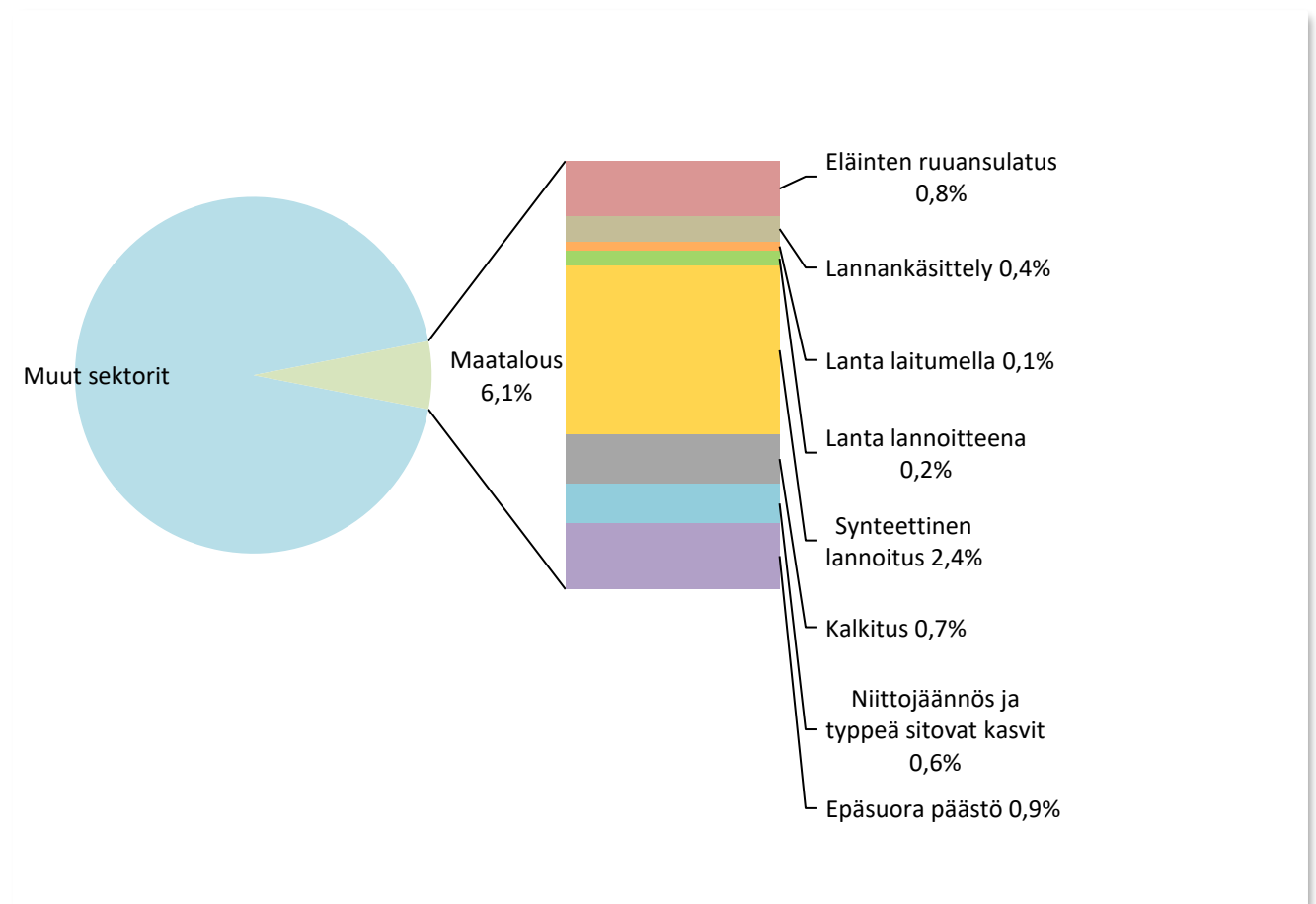
Kuva 9. Maatalouden päästöjen osuus kokonaispäästöistä (ilman teollisuutta) Karkkilassa vuonna 2016 ja sektorin jakautuminen eri päästölähteisiin.
