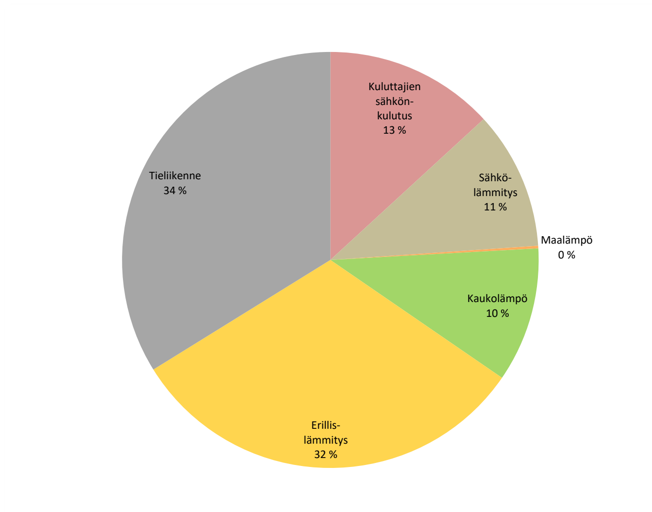
Kuva 13. Energian loppukulutuksen jakautuminen eri sektoreille Karkkilassa vuonna 2016 ilman teollisuutta. Energian loppukulutus ei sisällä lämpöpumppujen tuottamaa uusiutuvaa energiaa, mutta sisältää niiden käyttämän sähkön.
