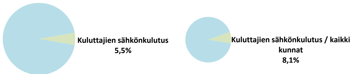
Kuva 2. Kuluttajien sähkönkulutuksen päästöjen osuus kokonaispäästöistä (ilman teollisuutta) Karkkilassa ja CO2-raportin kunnissa keskimäärin vuonna 2016.
