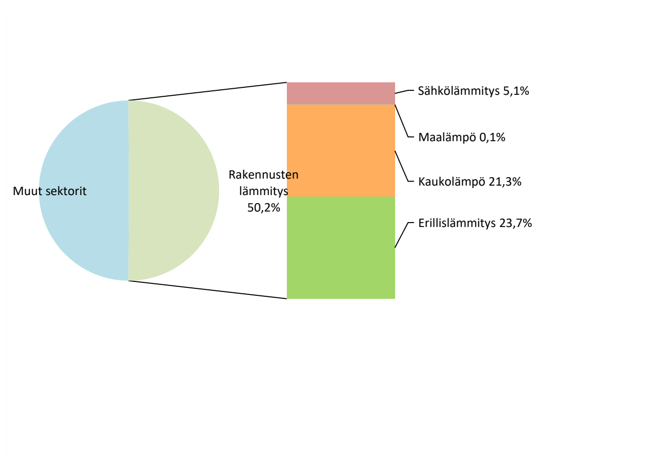
Kuva 5. Rakennusten lämmityksen päästöjen osuus kokonaispäästöistä (ilman teollisuutta) Karkkilassa vuonna 2016 ja sektorin jakautuminen eri päästölähteisiin.
