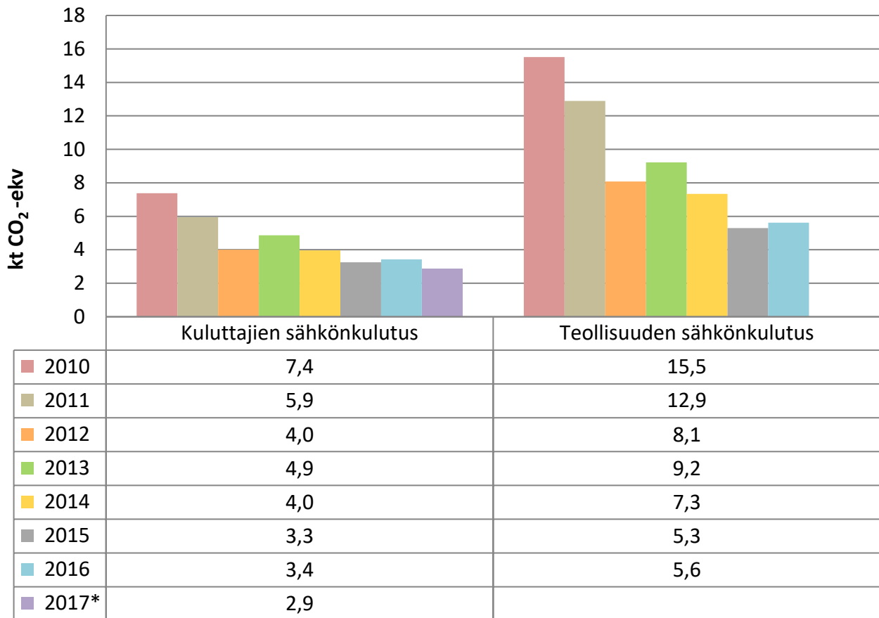
Kuva 3. Kuluttajien ja teollisuuden sähkönkulutuksen päästöjen kehitys Karkkilassa vuosina 2010–2017. Vuoden 2017 tieto on ennakkotieto. Sitä ei ole esitetty teollisuuden sähkönkulutukselle.
