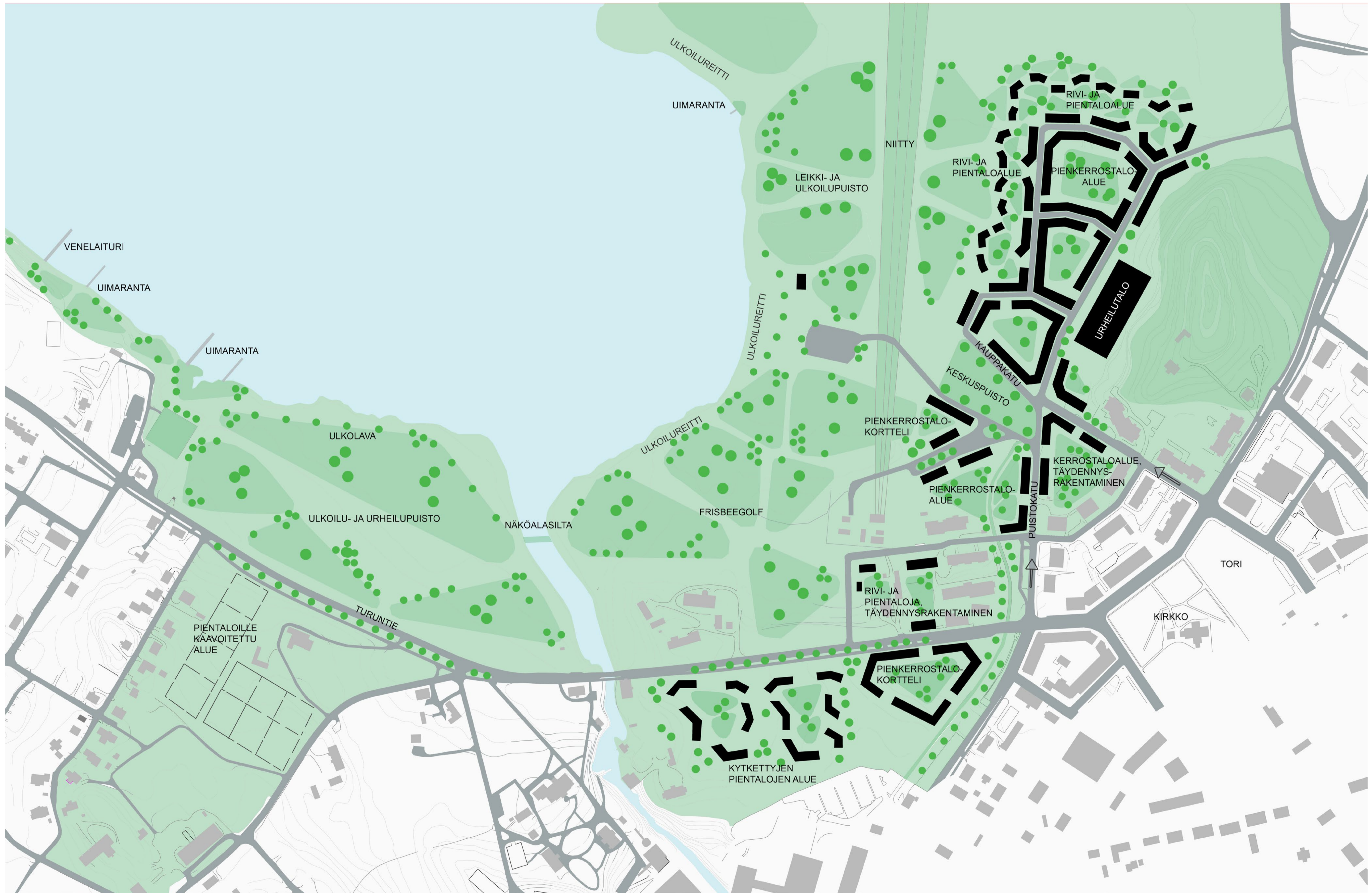
Yleissuunnitelma 1:2000
