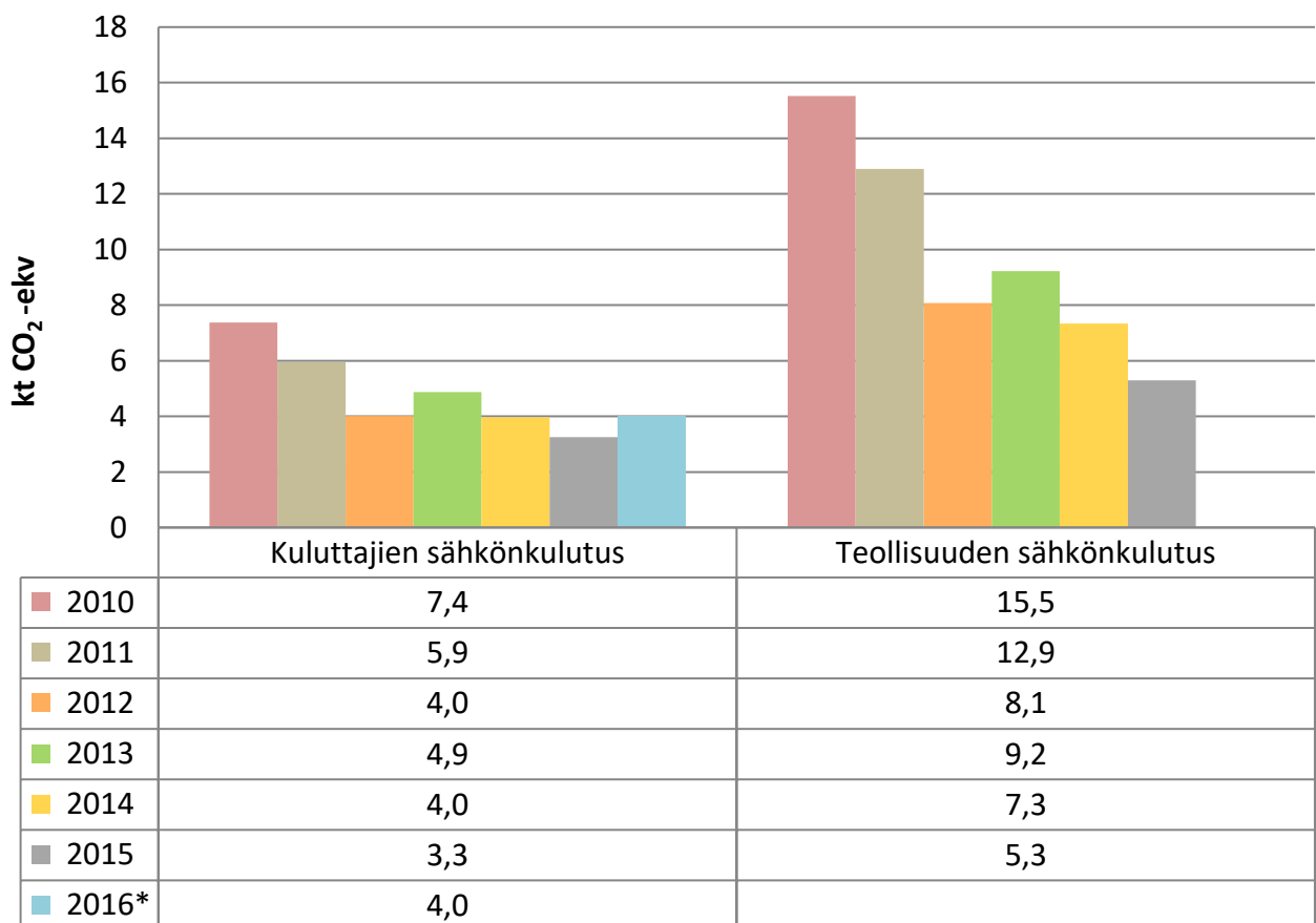
Kuva 3. Kuluttajien ja teollisuuden sähkönkulutuksen päästöjen kehitys Karkkilassa vuosina 2010–2016. Vuoden 2016 tieto on ennakkotieto. Sitä ei ole esitetty teollisuuden sähkönkulutukselle.
