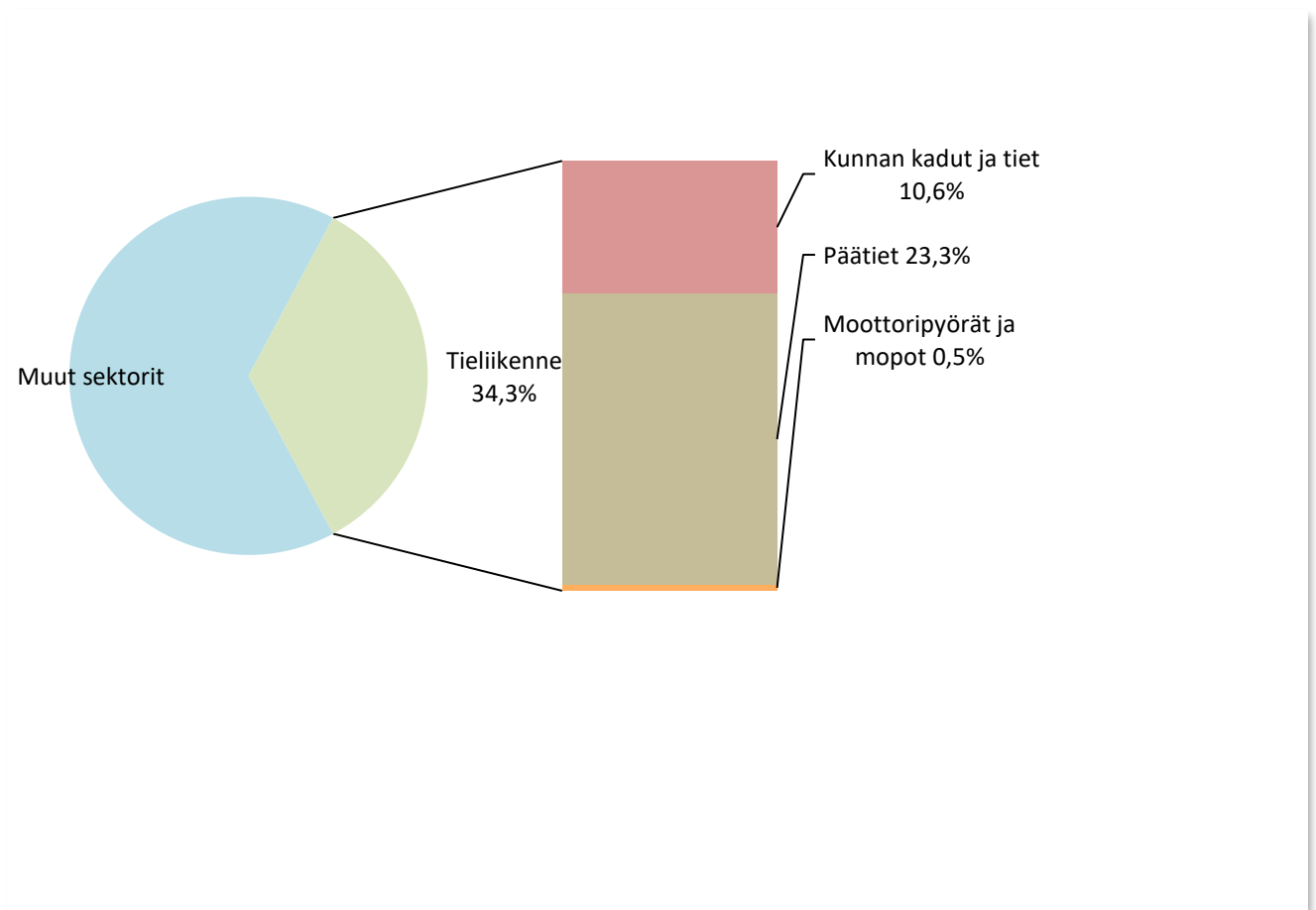
Kuva 7. Tieliikenteen päästöjen osuus kokonaispäästöistä (ilman teollisuutta) Karkkilassa vuonna 2015 ja sektorin jakautuminen eri päästölähteisiin.
