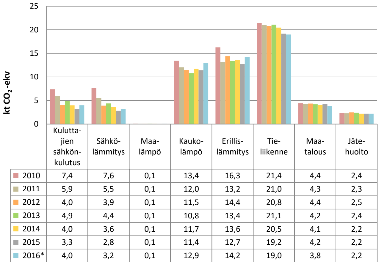
Kuva 15. Päästöt sektoreittain Karkkilassa vuosina 2010–2016 ilman teollisuutta. Vuoden 2016 tieto on ennakkotieto.
