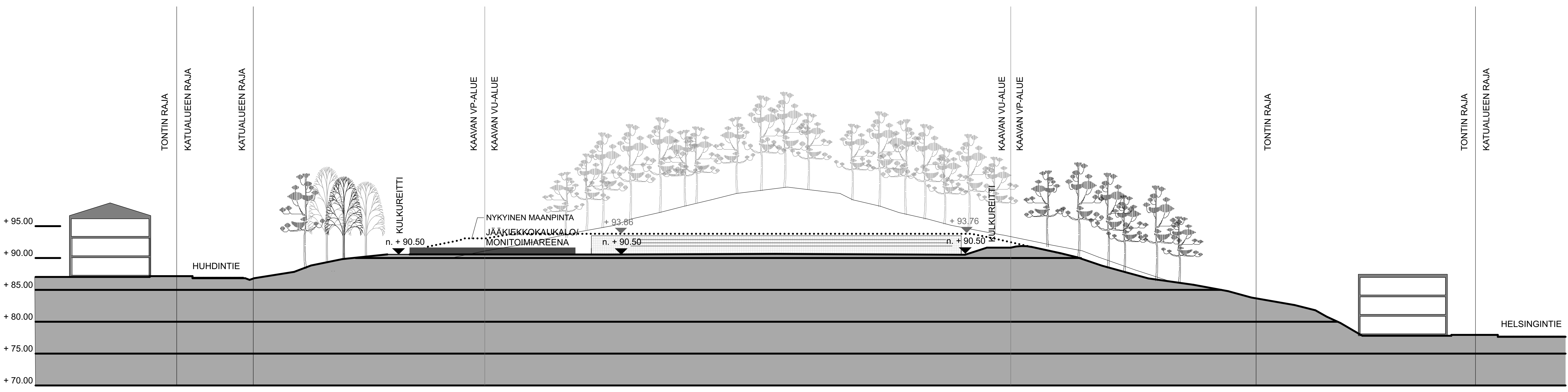
LEIKKAUS A-A 1:300
