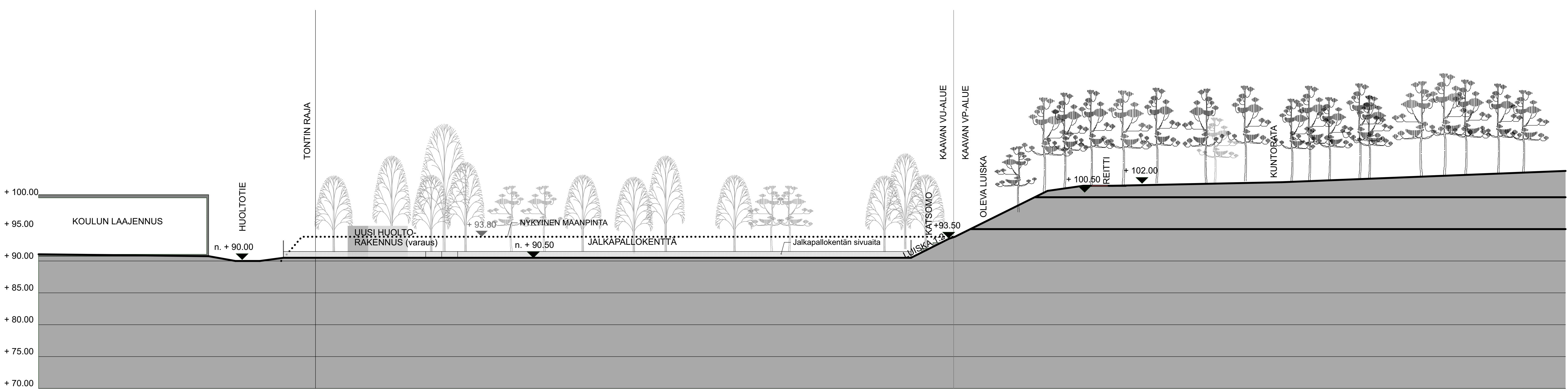
LEIKKAUS B-B 1:300
