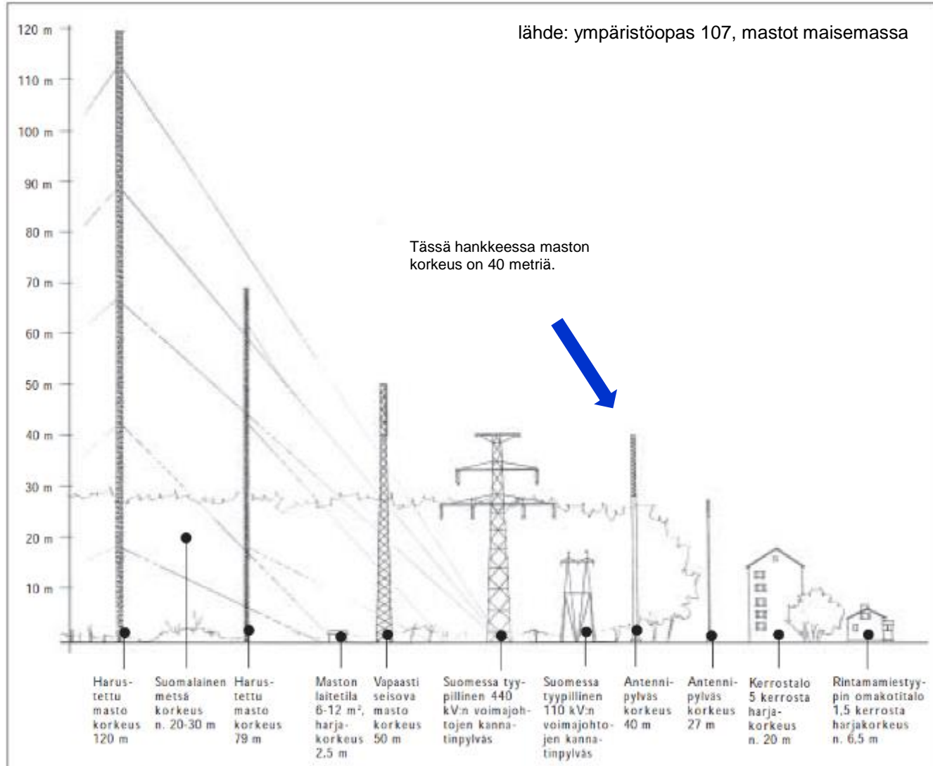
Kuva 1. Erilaisia mastotyyppjejä mittakaavallisessa vertailussa. Piirros Emilia Weckman.
